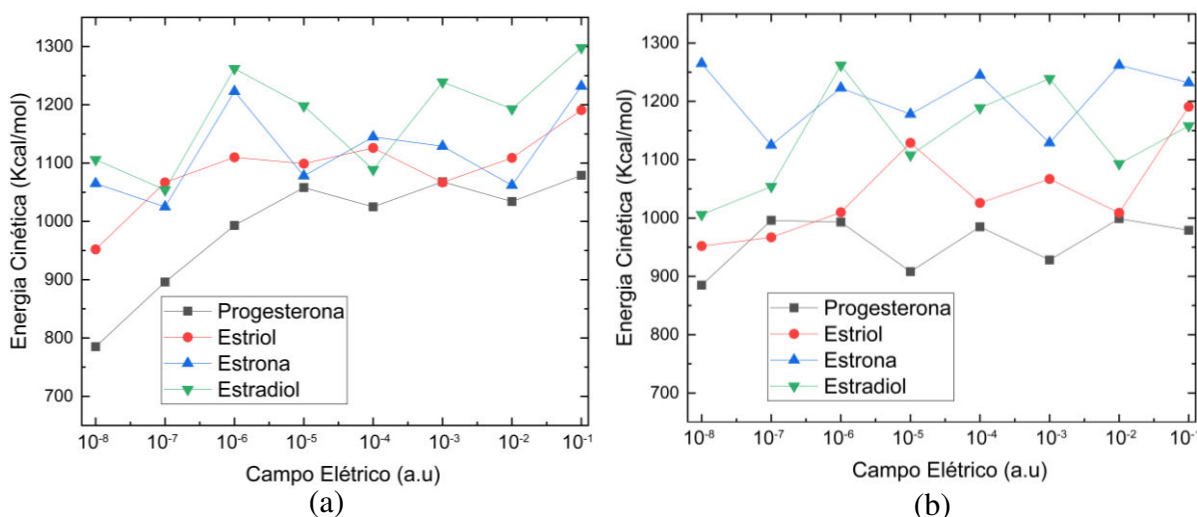
Figura 13: Energia cinética dos hormônios naturais na NF em: a) NTC e b) NTN.
